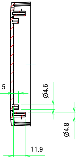
C-C (1:2)
